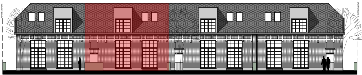
achtergevel
