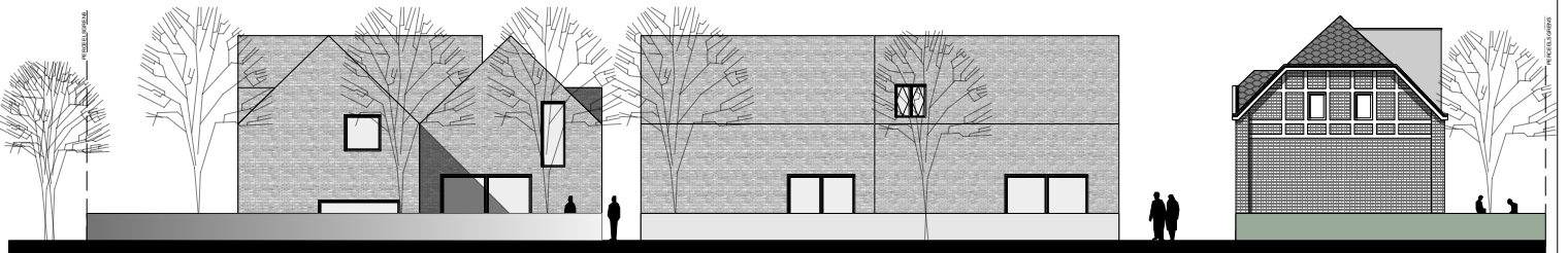
rechter zijgevel
