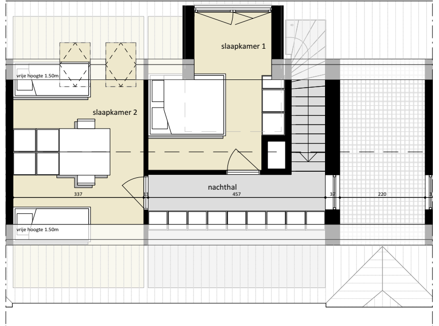
niveau +01
