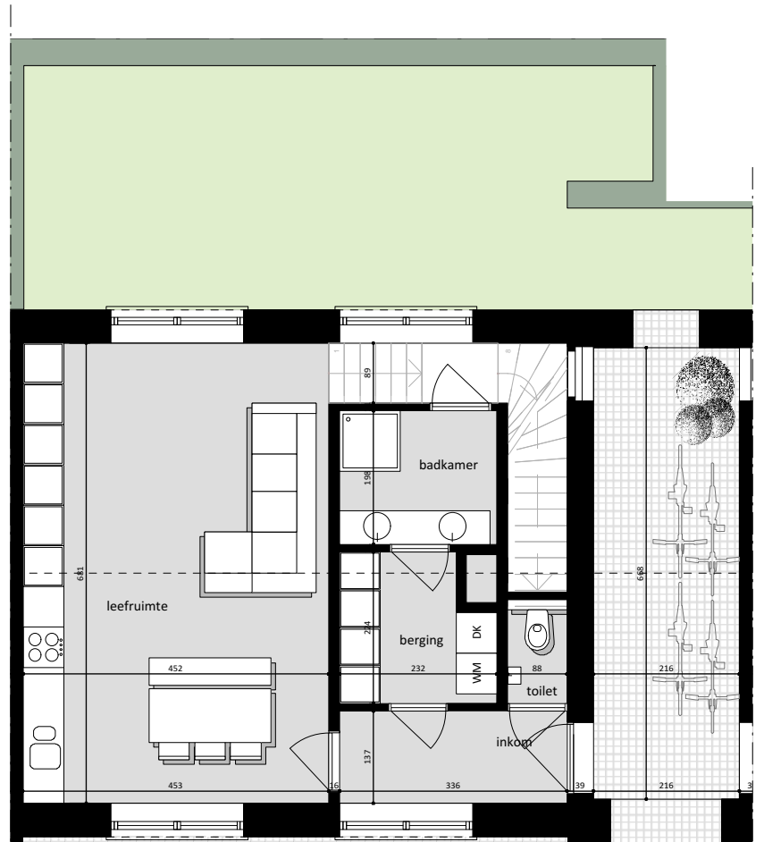
niveau 00
